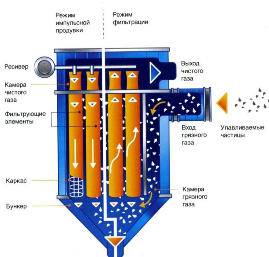
Рисунок 2.23 — Рукавный фильтр с импульсной регенерацией.
