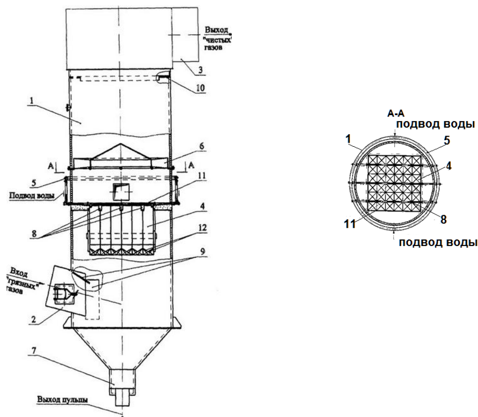
Рисунок 2.11 — Батарейный эмульгатор:
