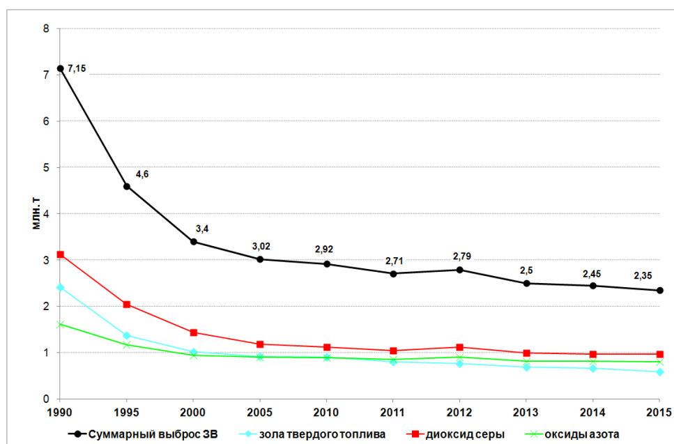
Рисунок 1.9 — Выбросы загрязняющих веществ ТЭС отрасли электроэнергетика
