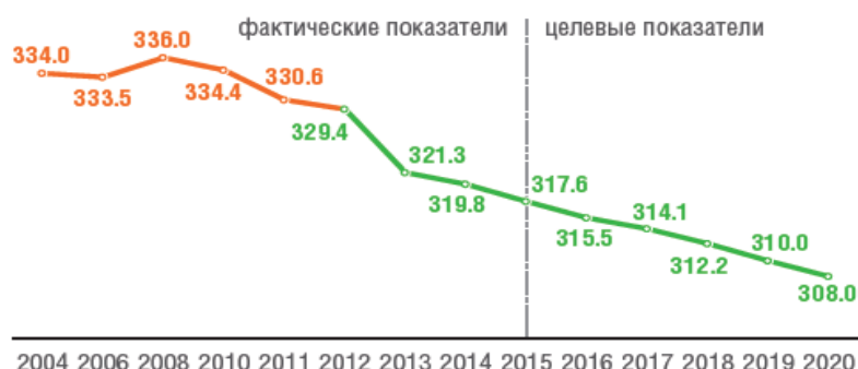
Рисунок 1.8 – Удельный расход условного топлива на отпуск электрической энергии (пропорциональный метод), г/кВт*ч [18]
