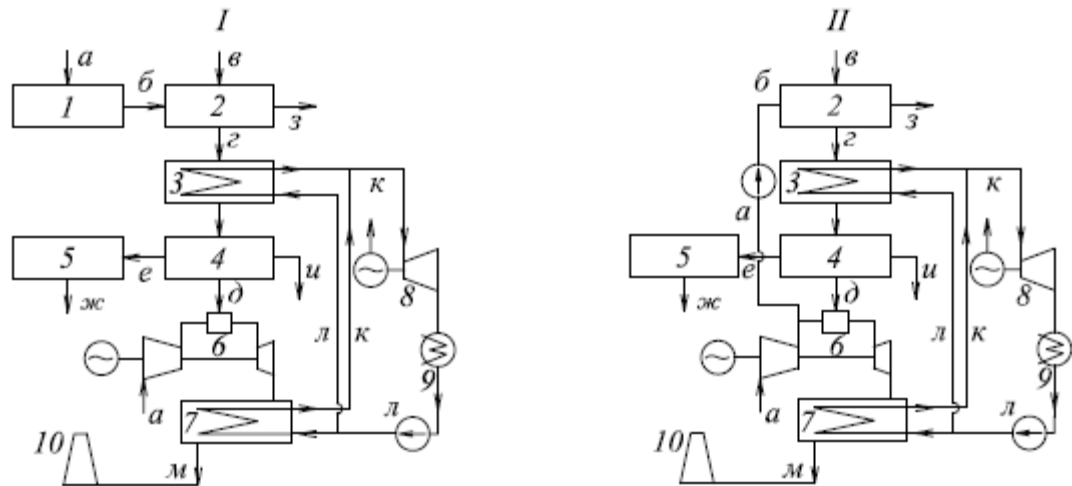
Рисунок 2.18 – Принципиальные схемы ПГУ:
