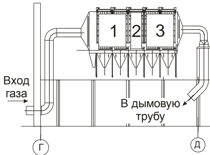
Рисунок 2.20 — Принципиальная схема комбинированного золоуловителя
