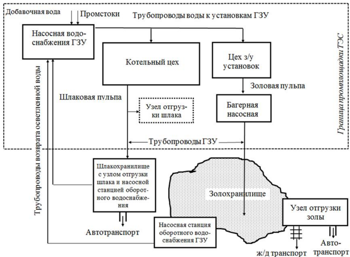
Рисунок 2.14 — Блок-схема системы ГЗУ с разделением удалением, складированием и отгрузкой золы и шлака
