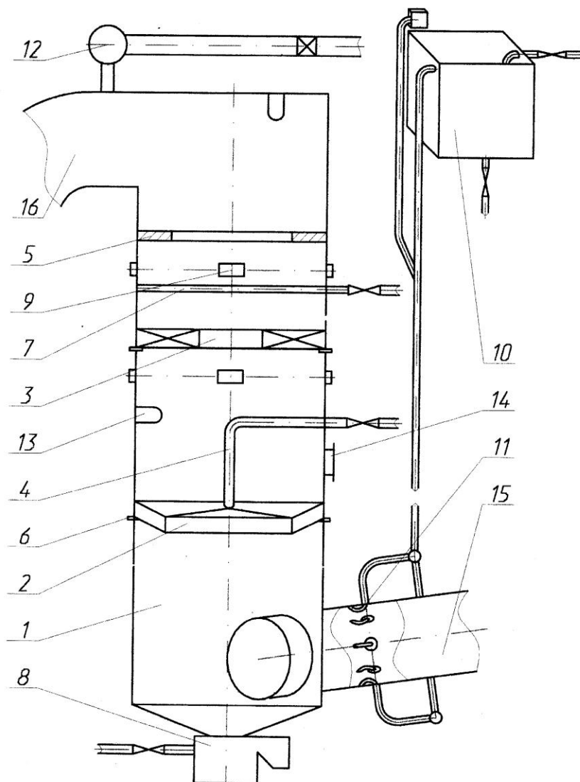
Рисунок 2.12. — Кольцевой эмульгатор
