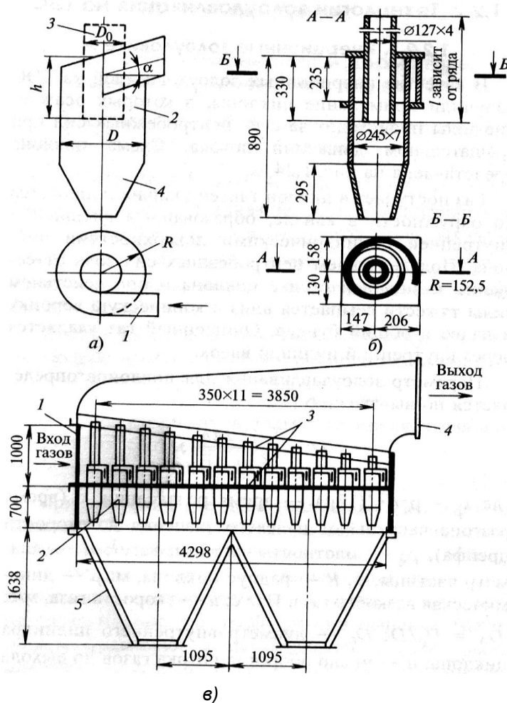
Рисунок 2.10 — Циклонные золоуловители
