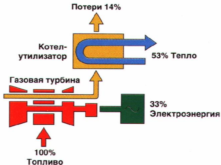
Рисунок 3.2 — Схема ГТУ-ТЭЦ
