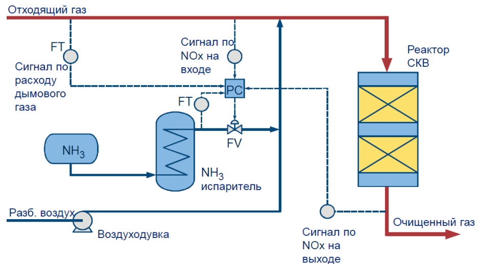
Рисунок 2.25 — Схема установки СКВ с применением аммиака
