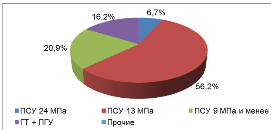
Рисунок 1.4 — Структура генерирующих мощностей ТЭС с разбивкой по параметрам и составу оборудования
