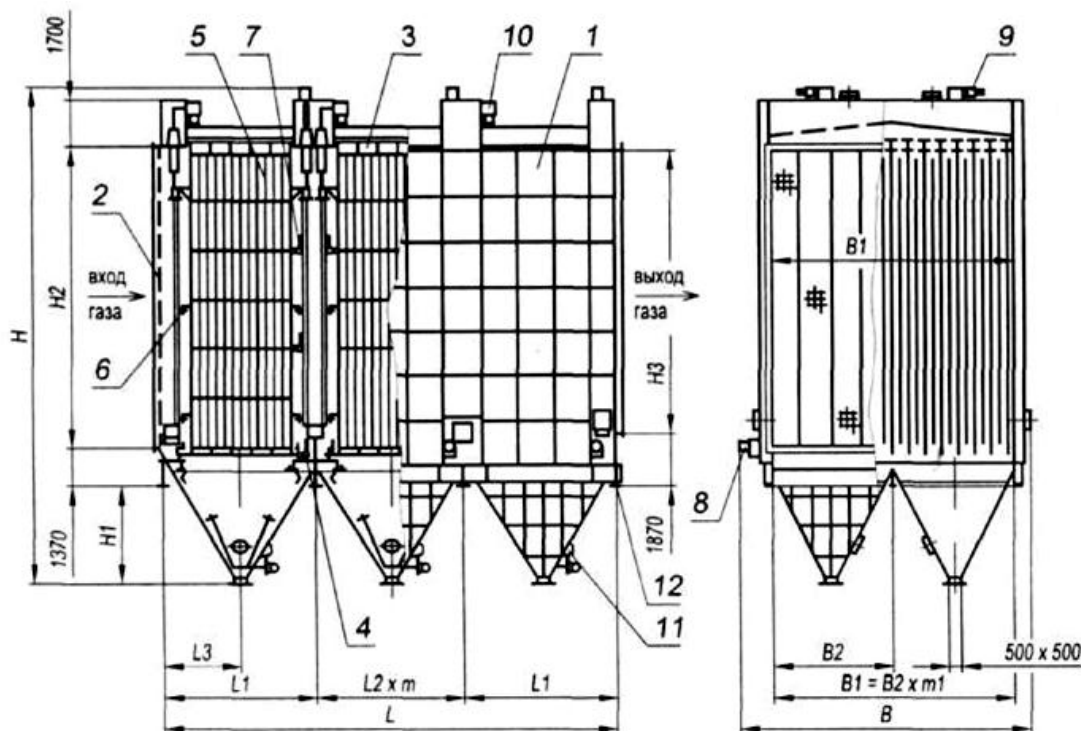
Рисунок 2.8 — Двухсекционный трехполюсный электрофильтр
